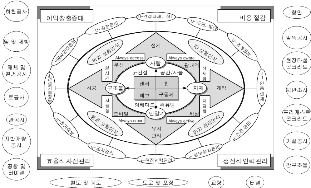
[그림 4-11] 유비쿼터스 건설 프로세스 모형(예시)
