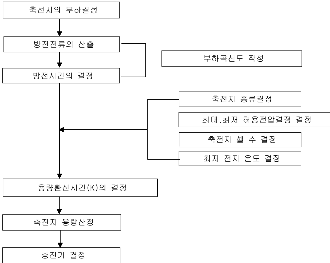
[그림 3-15] 축전기 및 충전기 용량 산정 절차
